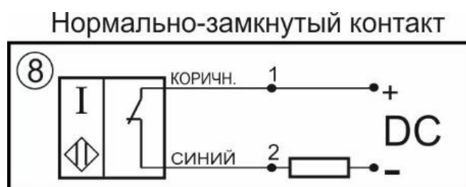
Схема соединения
