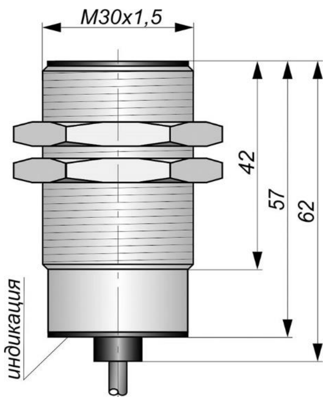
Габаритный чертеж
