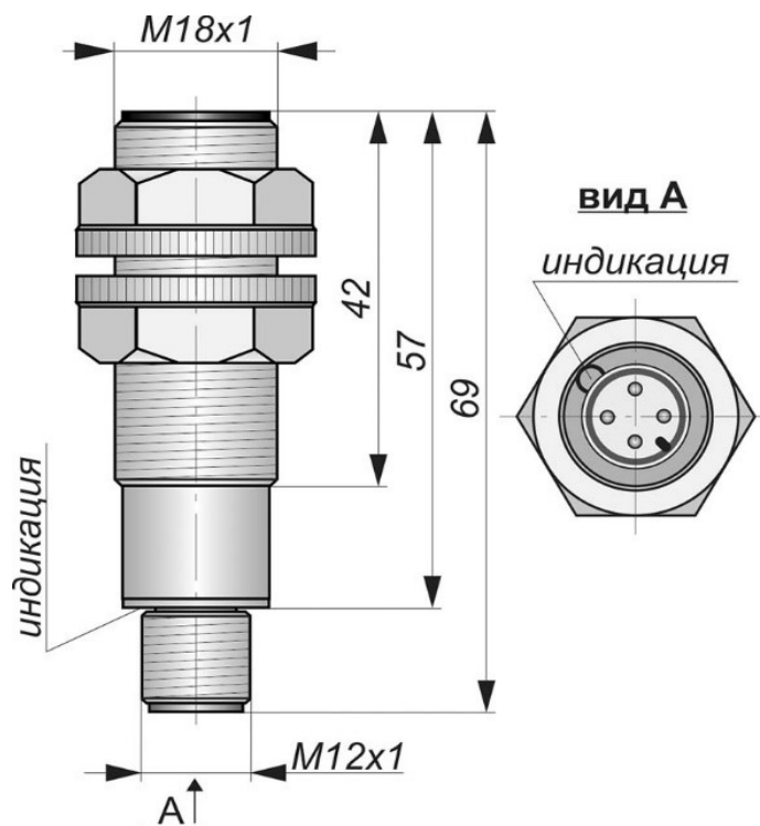
Габаритный чертеж
