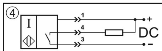
Цоколевка разъема
