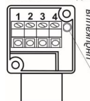
Цоколевка клеммной колодки
