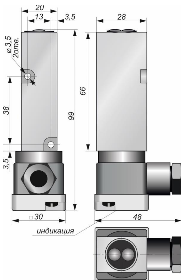
Габаритный чертеж
