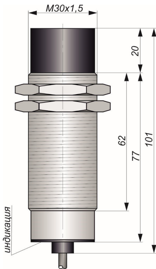
Габаритный чертеж
