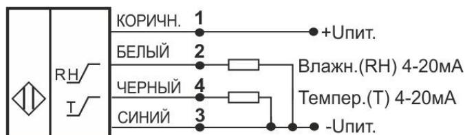
Схема подключения
