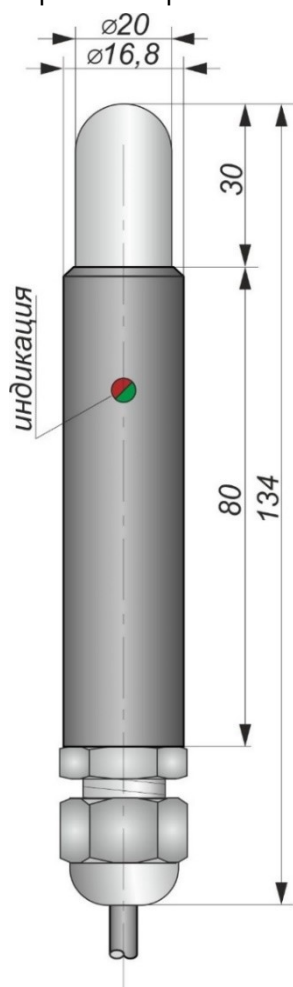
Габаритный чертеж
