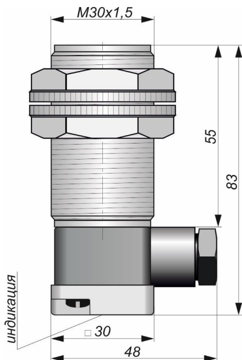
Габаритный чертеж
