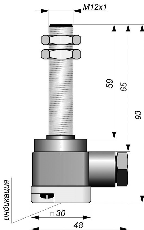
Габаритный чертеж
