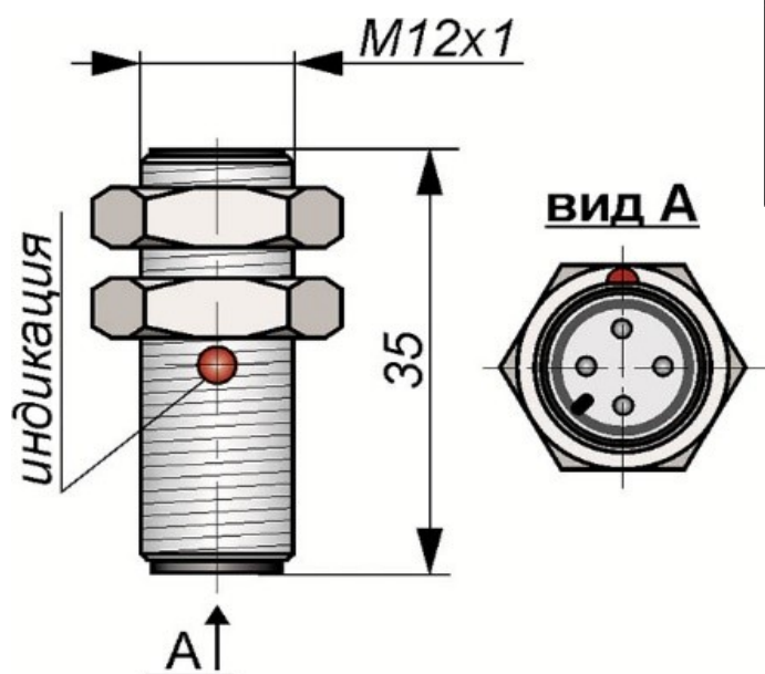
Габаритный чертеж
