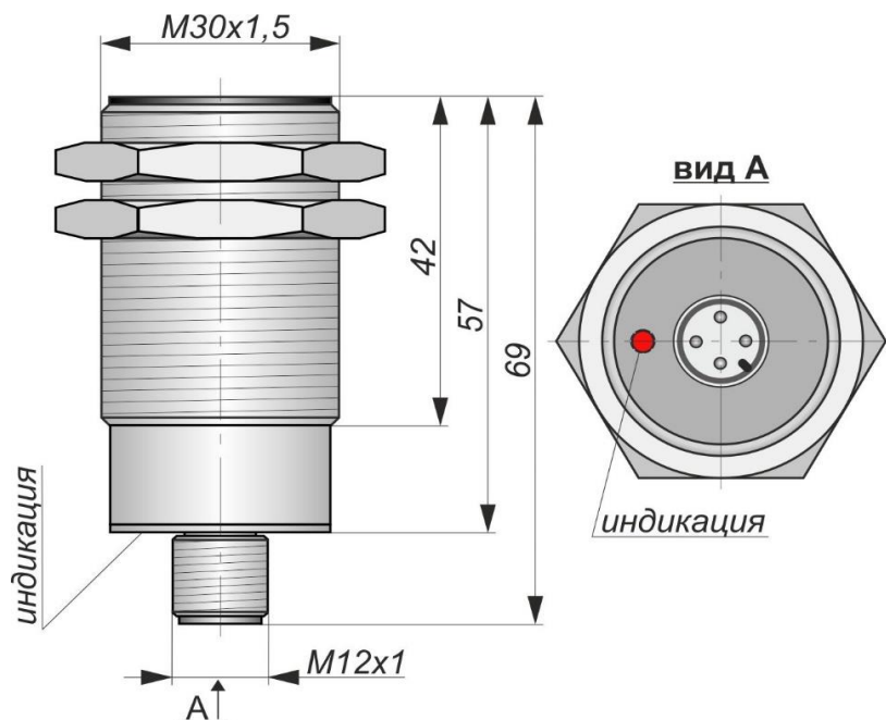
Габаритный чертеж
