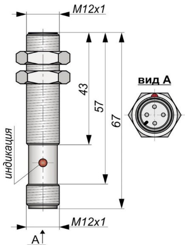
Габаритный чертеж
