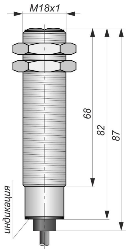
Габаритный чертеж
