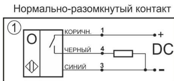
Схема соединения
