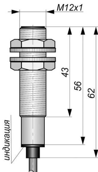
Габаритный чертеж
