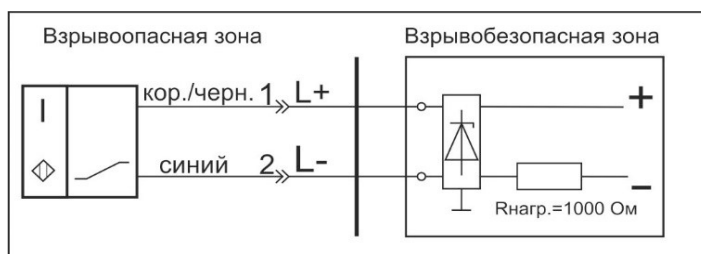
Схема соединения
