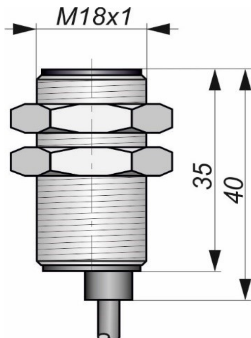
Габаритный чертеж
