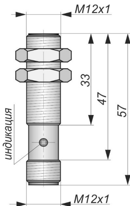
Габаритный чертеж
