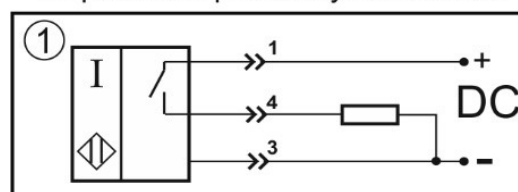
Цоколевка разъема
