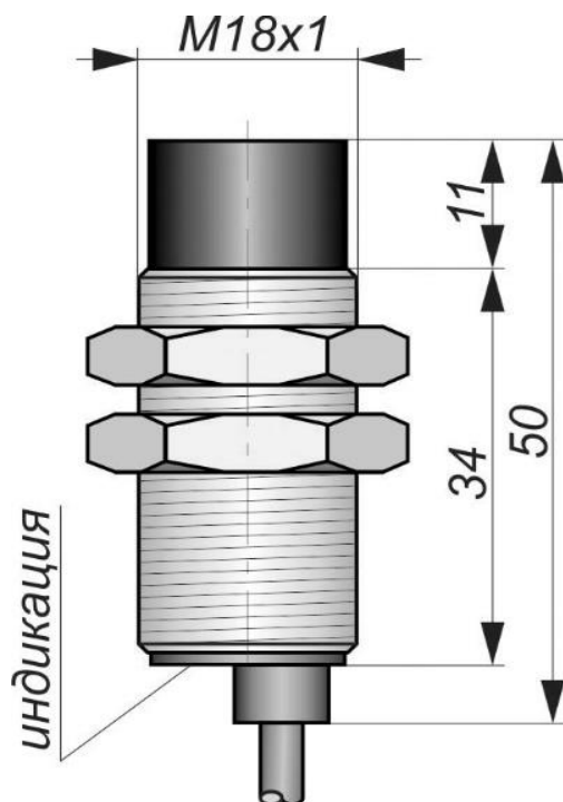
Габаритный чертеж
