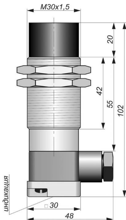
Габаритный чертеж
