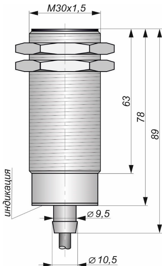
Габаритный чертеж
