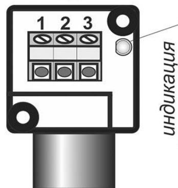
Цоколевка клеммной колодки
