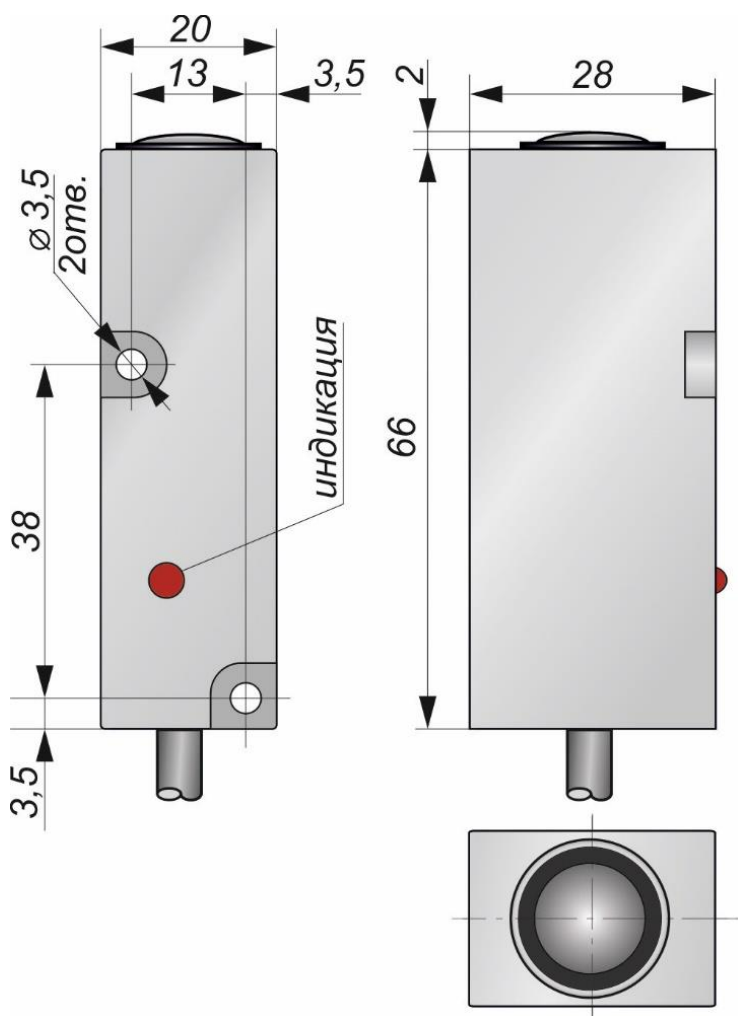
Габаритный чертеж
