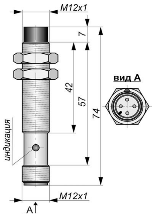
Габаритный чертеж
