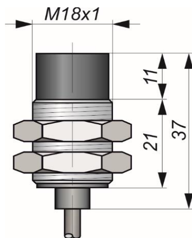
Габаритный чертеж
