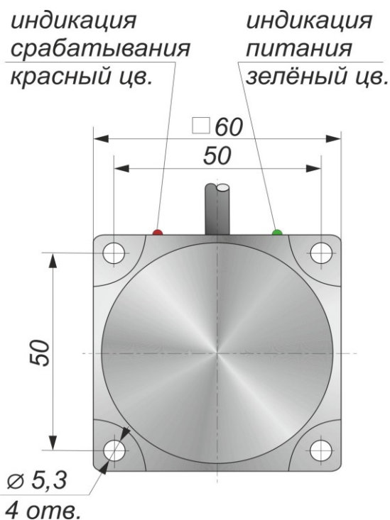
Габаритный чертеж
