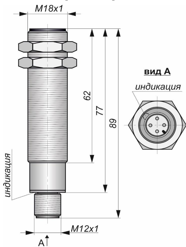
Габаритный чертеж
