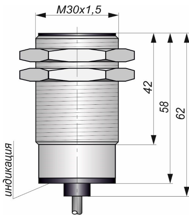
Габаритный чертеж
