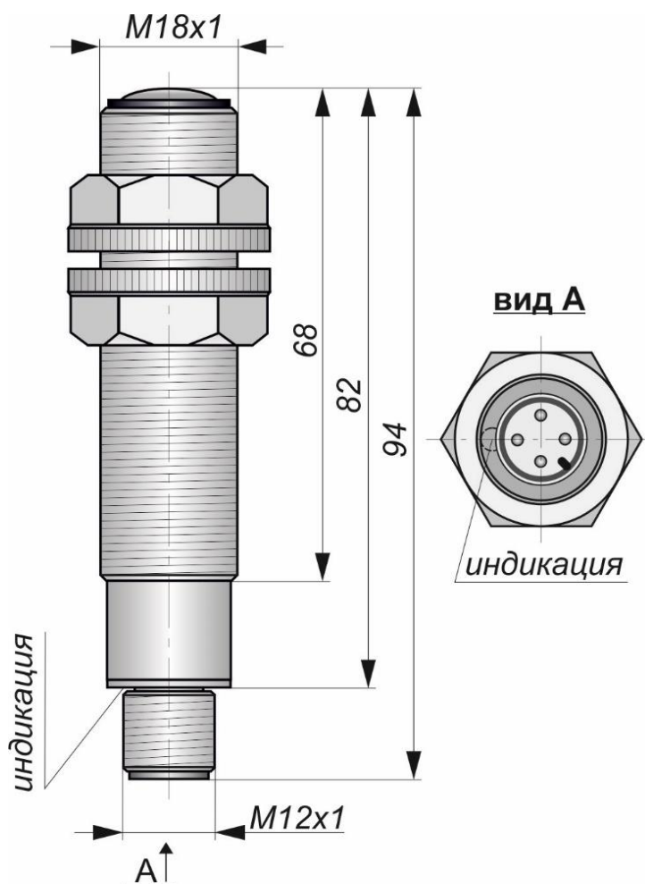
Габаритный чертеж
