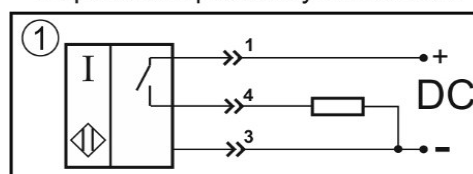
Цоколевка разъема
