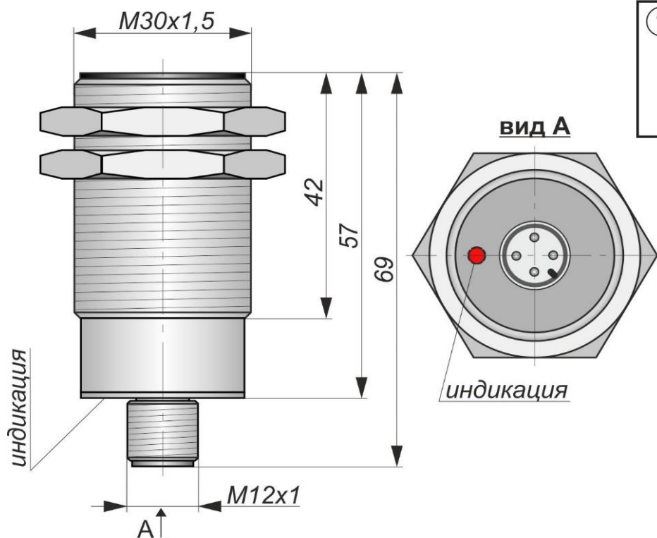
Габаритный чертеж
