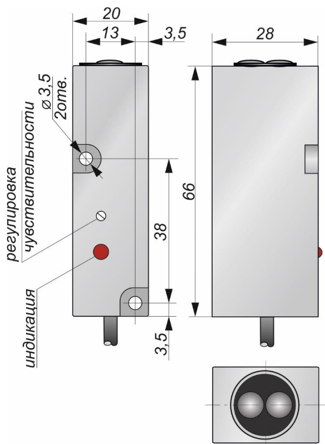
Габаритный чертеж
