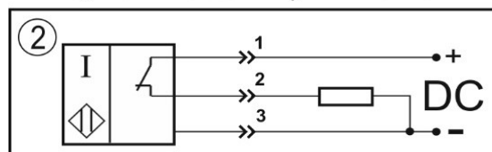
Цоколевка разъема
