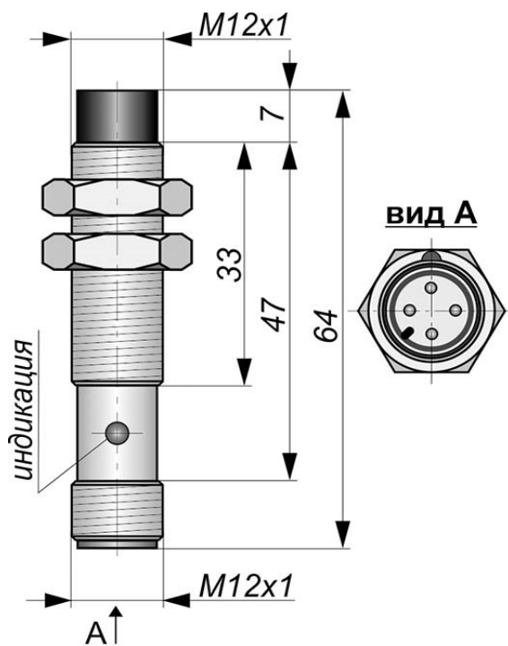
Габаритный чертеж
