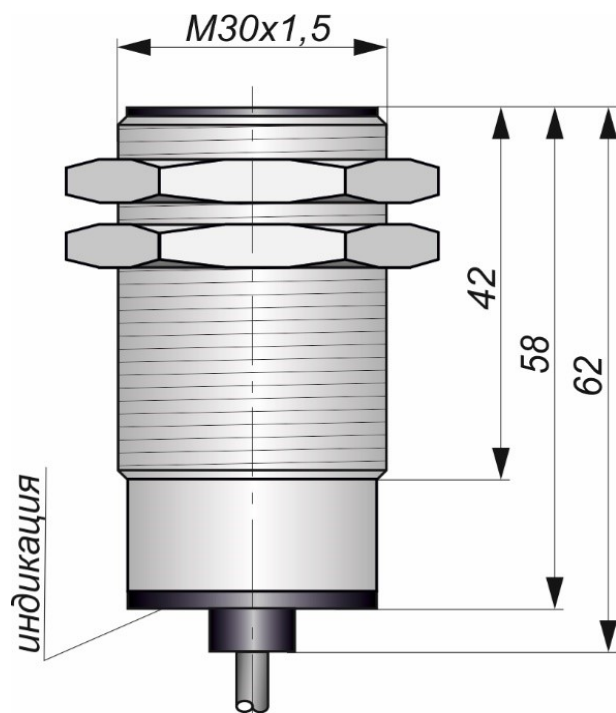
Габаритный чертеж
