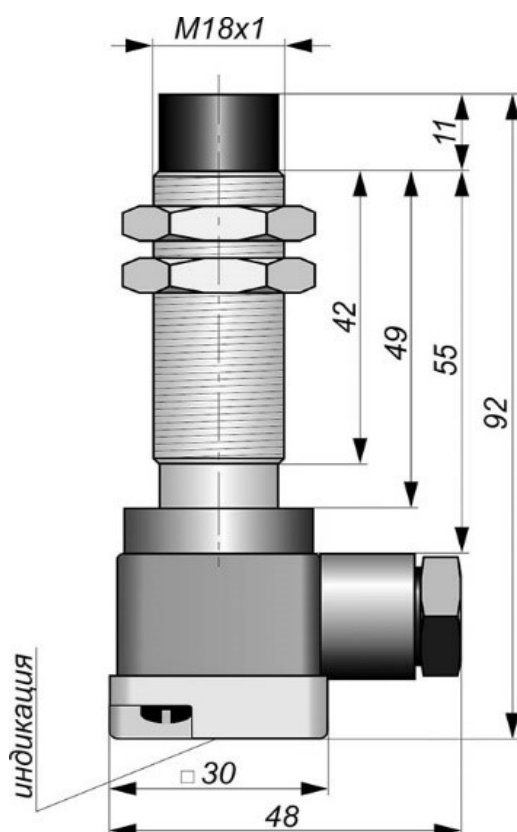
Габаритный чертеж
