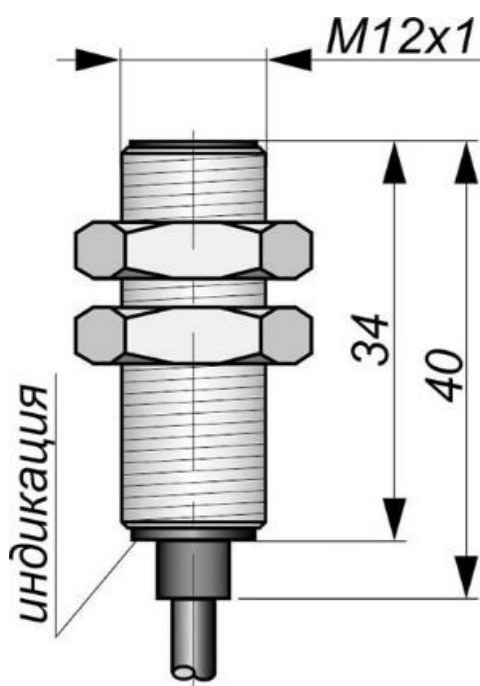
Габаритный чертеж
