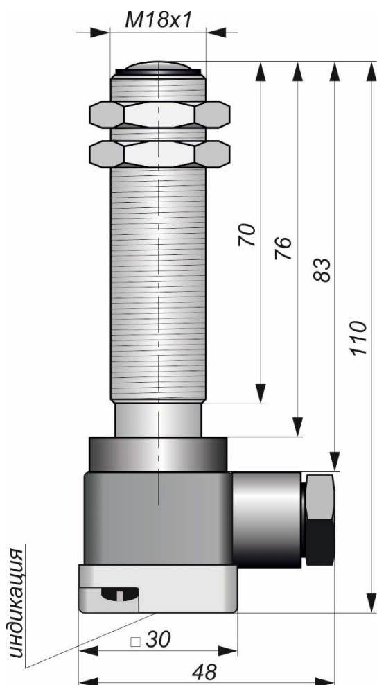
Габаритный чертеж
