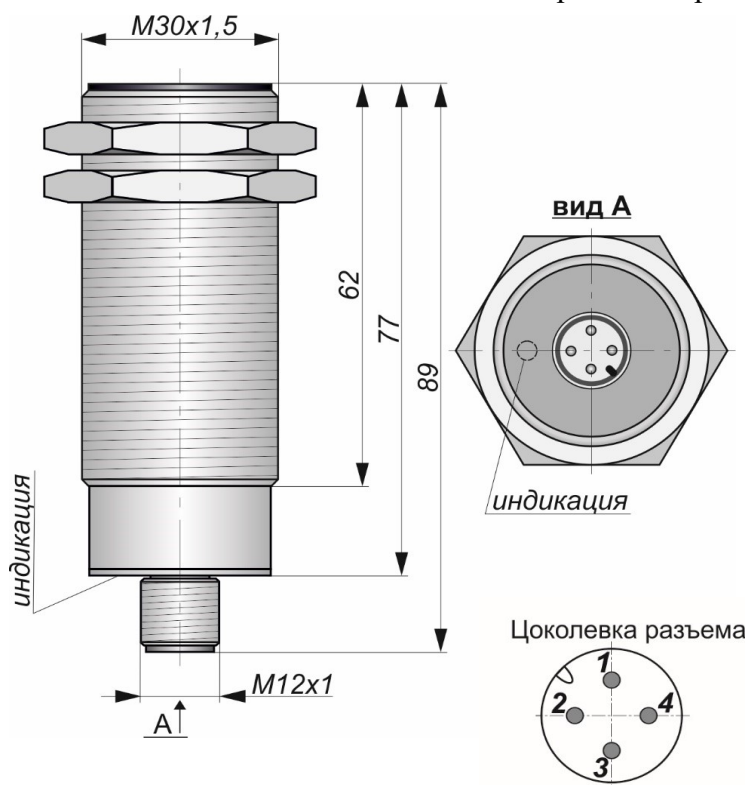
Габаритный чертеж
