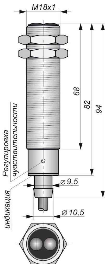
Габаритный чертеж
