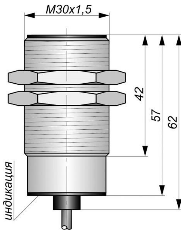
Габаритный чертеж
