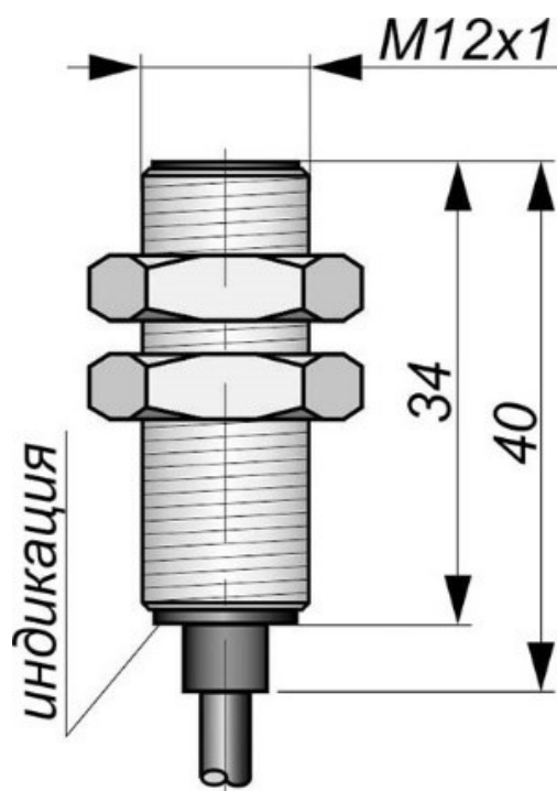
Габаритный чертеж
