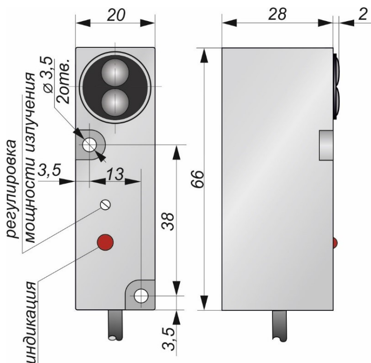
Габаритный чертеж
