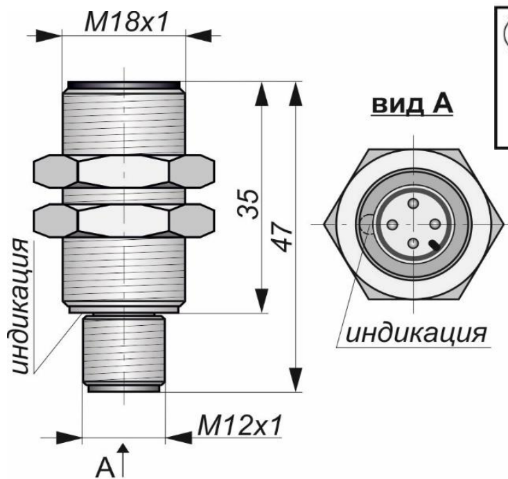
Габаритный чертеж
