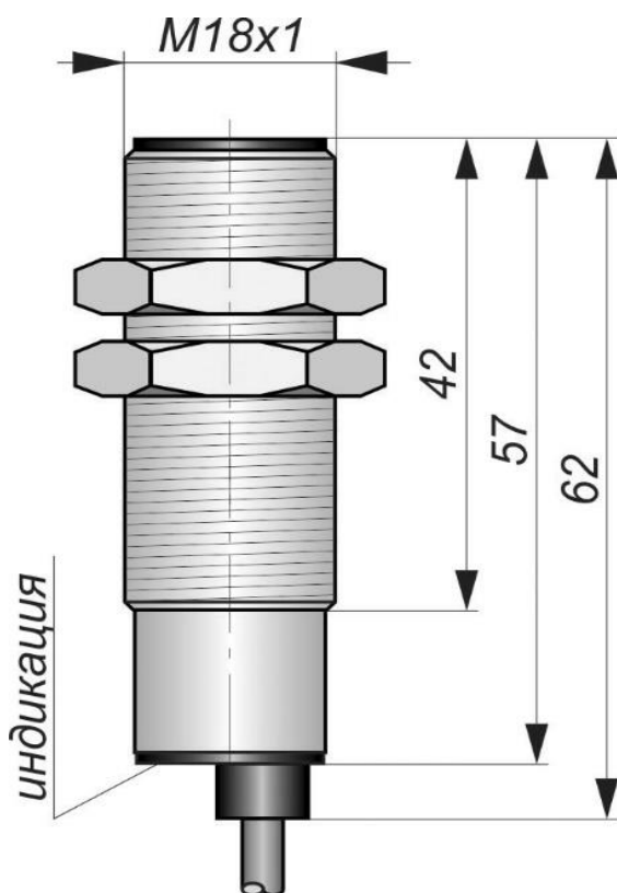
Габаритный чертеж
