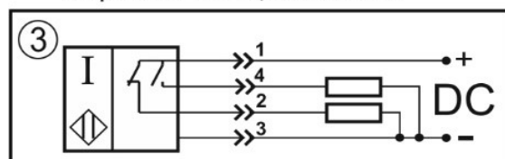
Переключающий контакт
