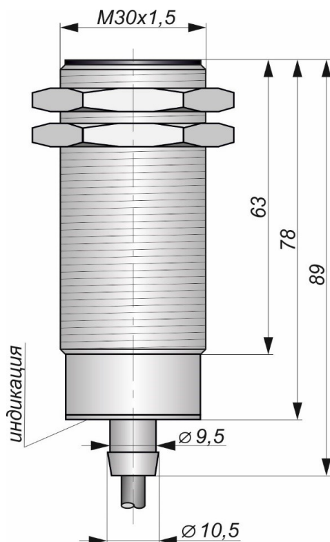
Габаритный чертеж
