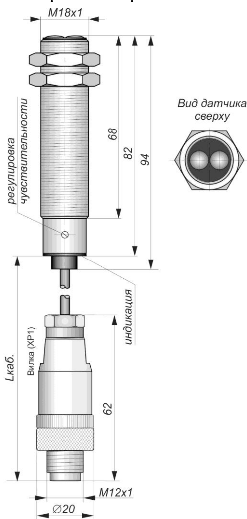
Габаритный чертеж
