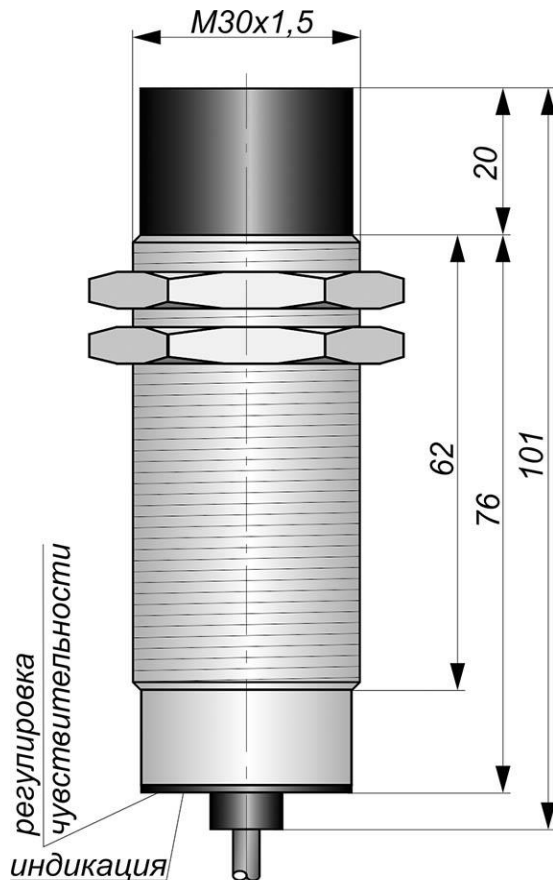
Габаритный чертеж
