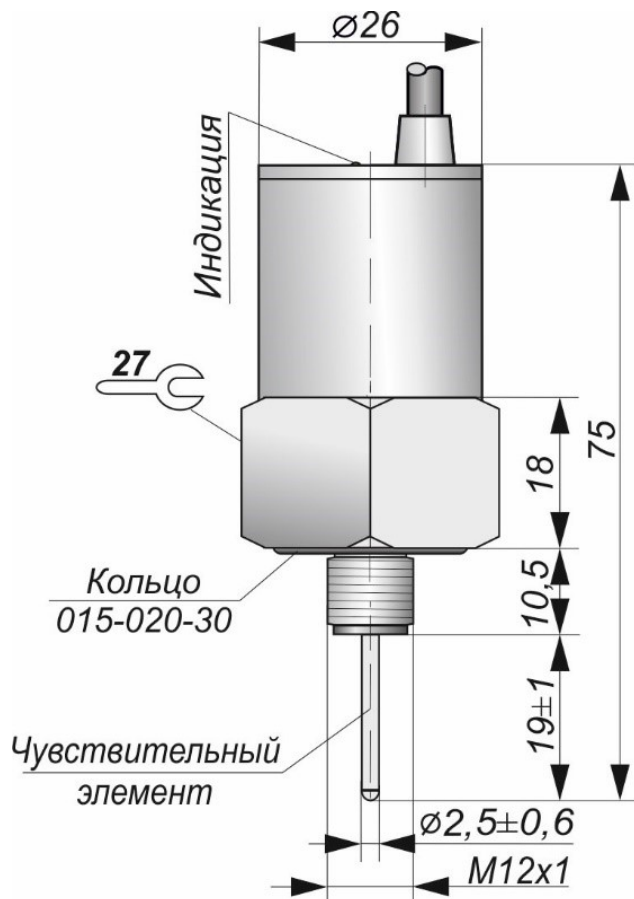
Габаритный чертеж
