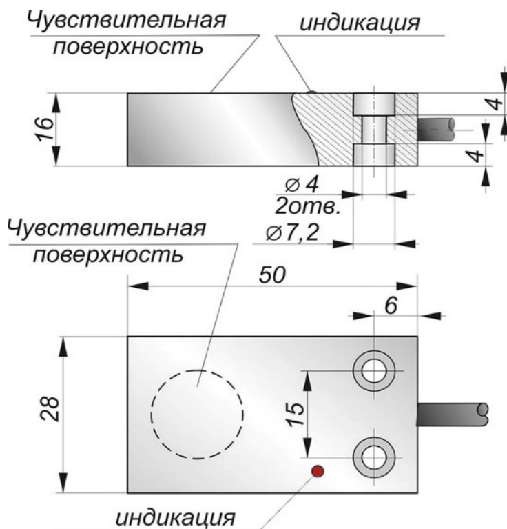
Габаритный чертеж
