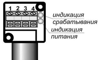
Цоколевка клеммной колодки
