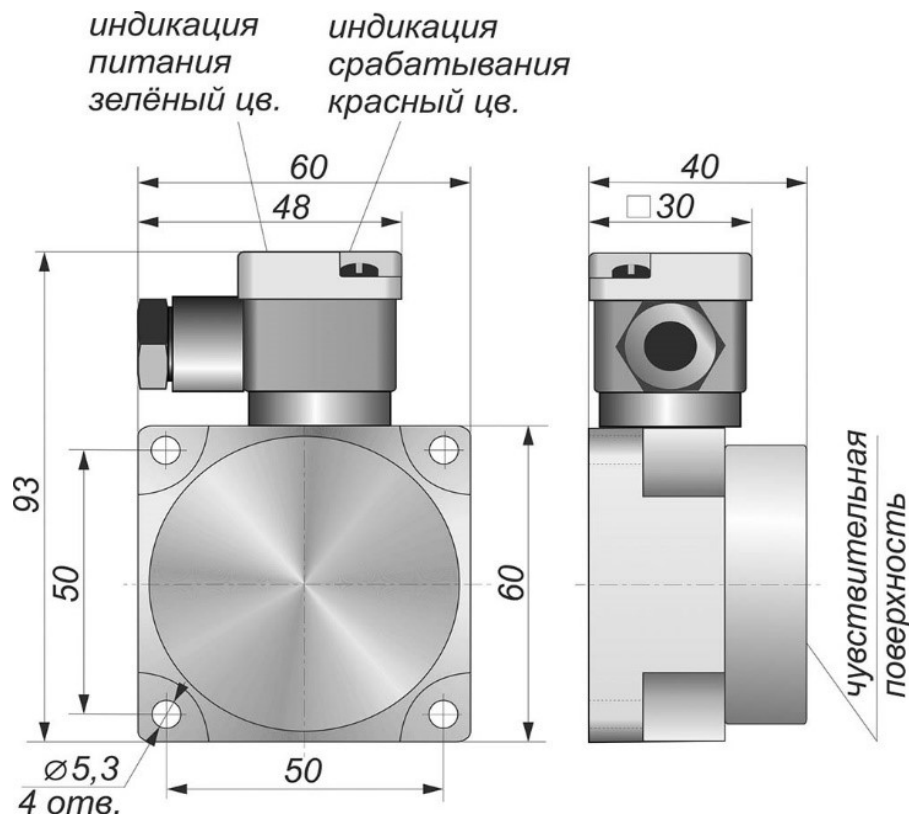
Габаритный чертеж
