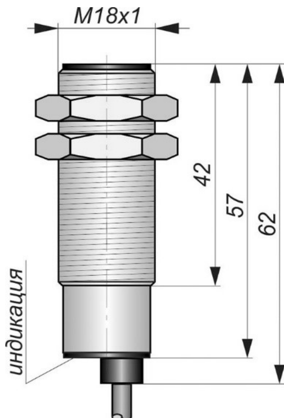
Габаритный чертеж
